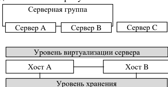
Рисунок 1 - Серверная архитектура
